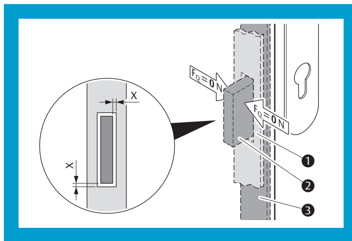
Fig. 8 : Pêne dormant exempt de contraintes transversales ( F_Q )
