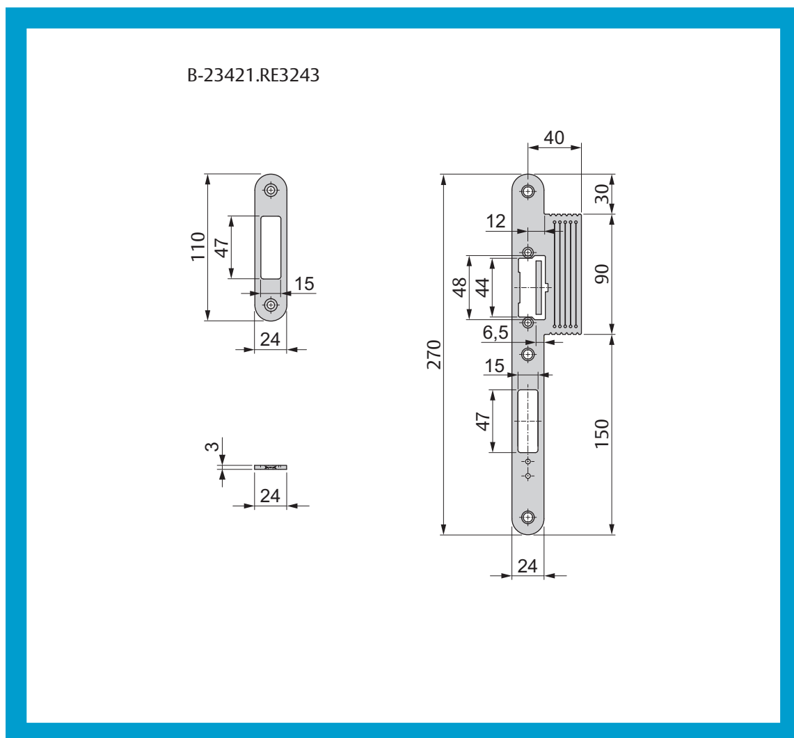
Fig. 8 : Têtières pour bois
