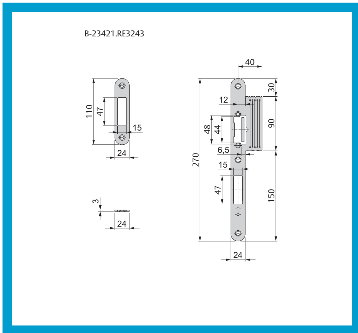
Fig. 8: Contropiastre per legno
